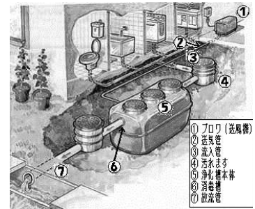
合併処理浄化槽イメージ図
